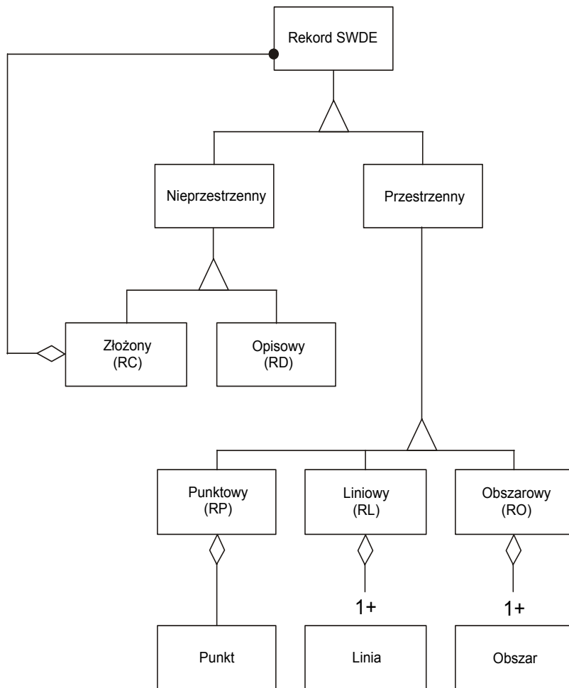
Rysunek 4. Struktura pliku danych SWDE
