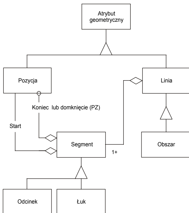
Rysunek 6. Atrybuty geometryczne obiektów przestrzennych w SWDE
